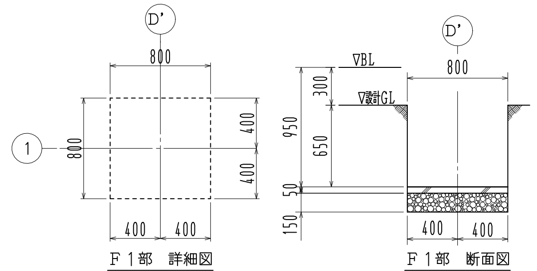
基礎詳細図 1/30
