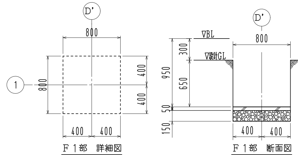
基礎詳細図 1/30
