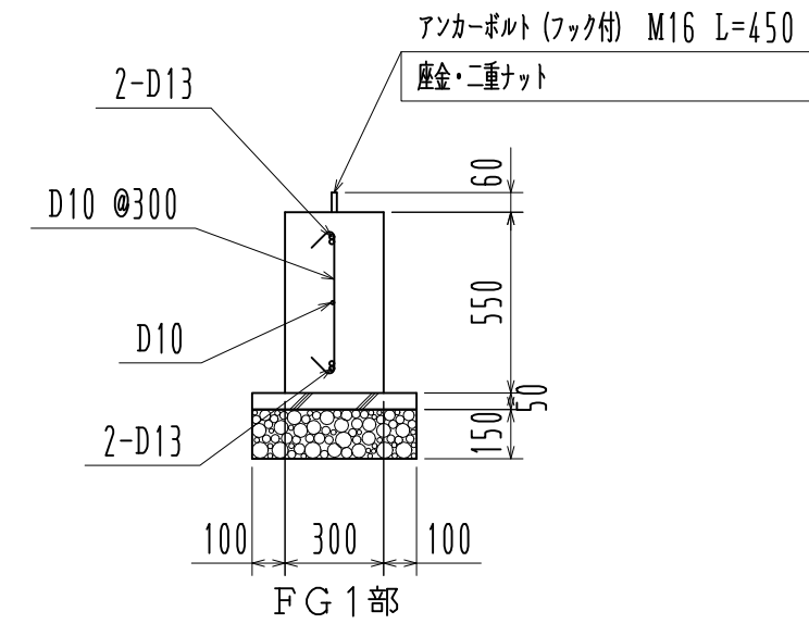
基礎詳細図 1/25
