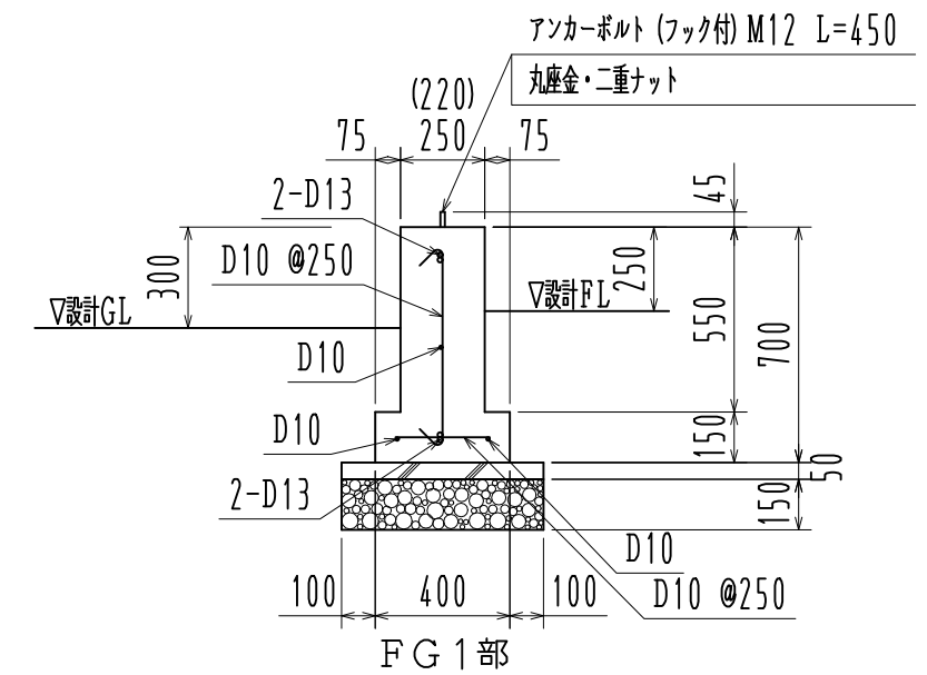
基礎詳細図 1/25
