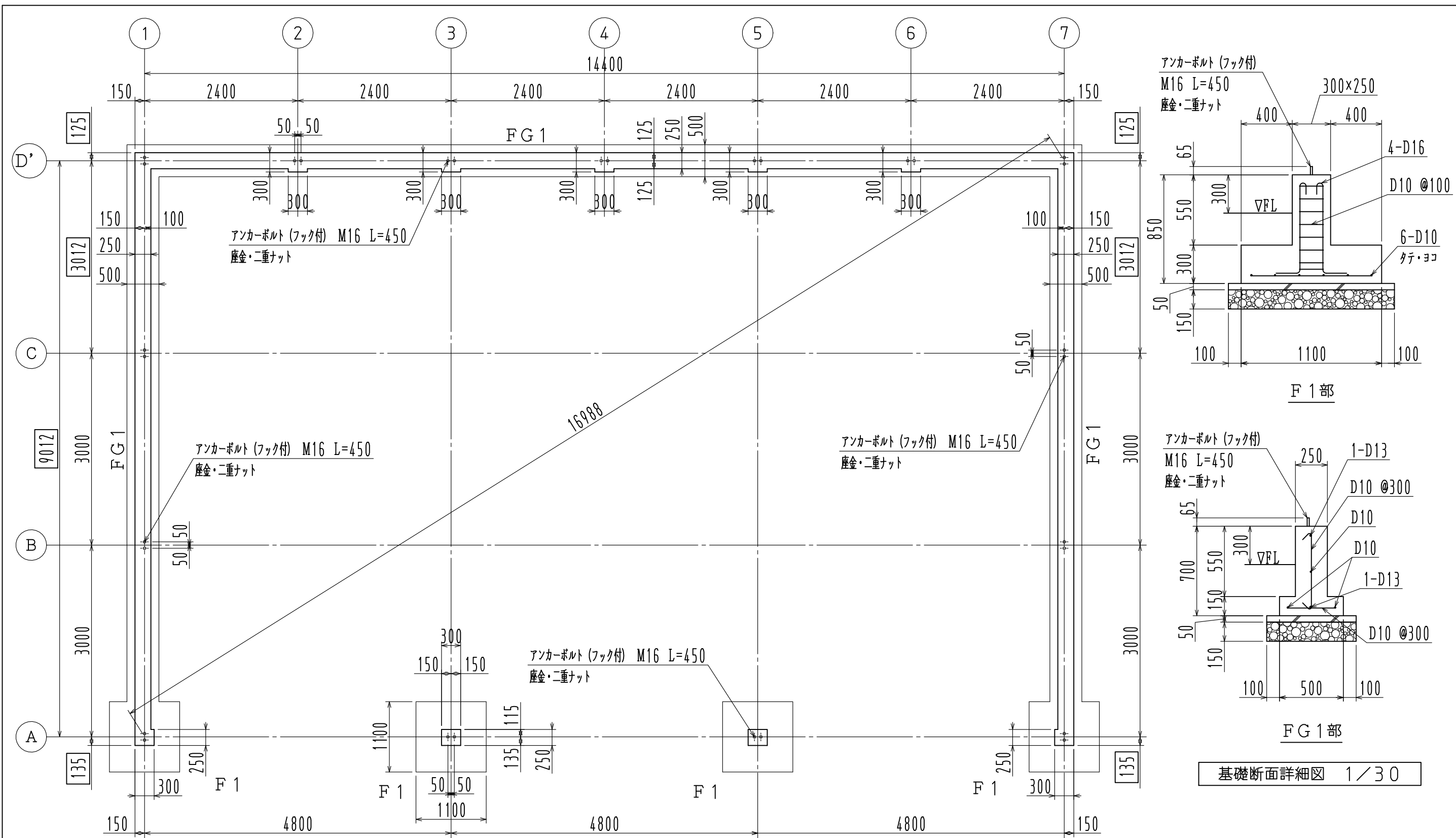
基礎伏図 1/60
