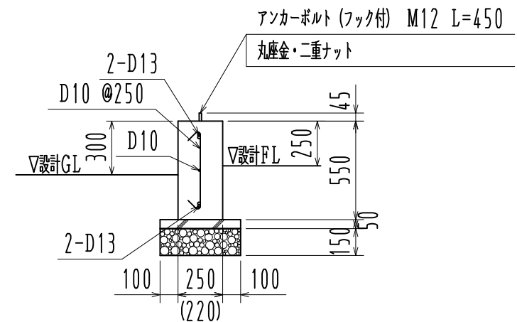
基礎詳細図 1/30
