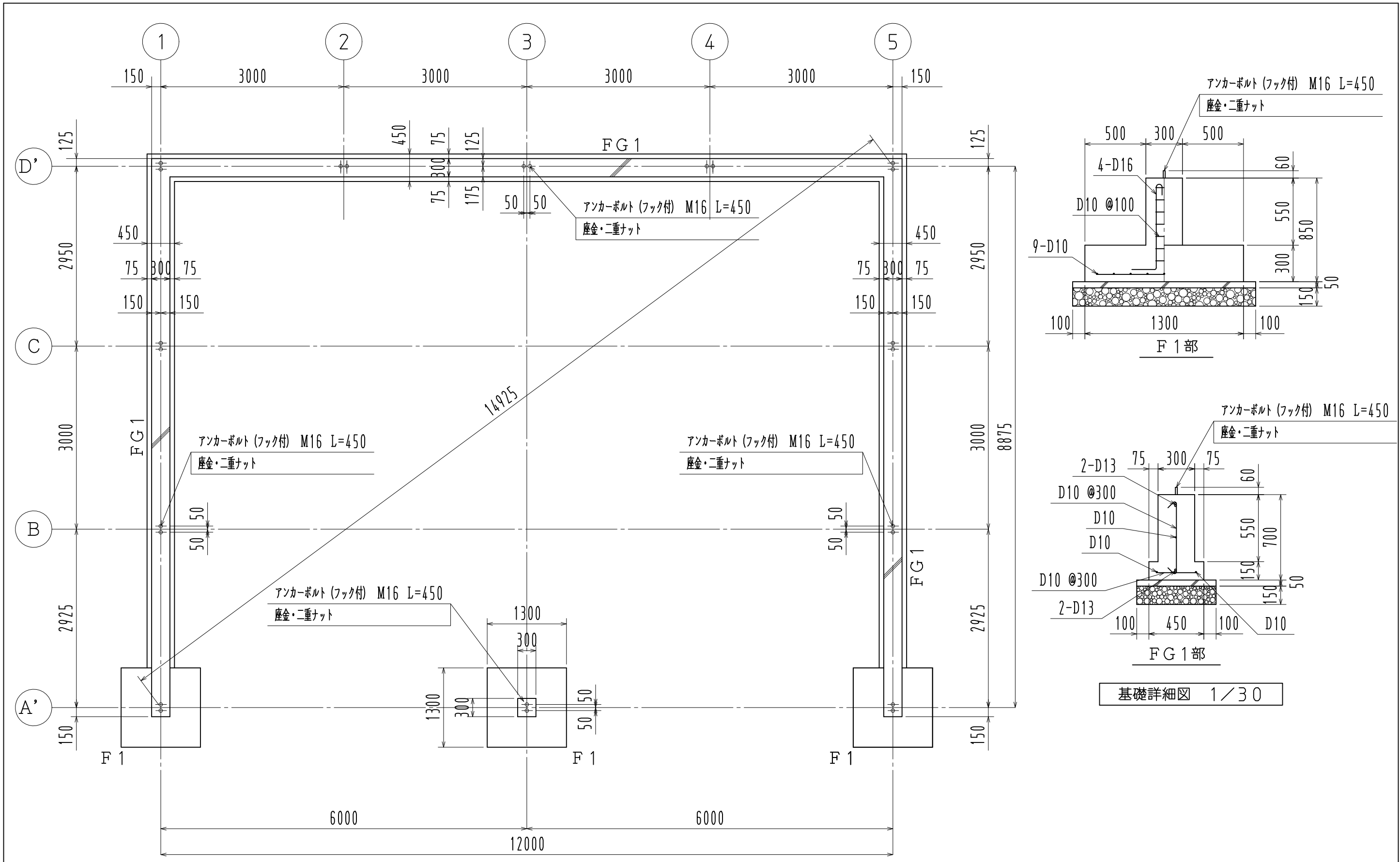
基礎伏図 1/60
