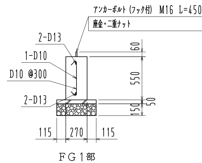
基礎詳細図 1/30
