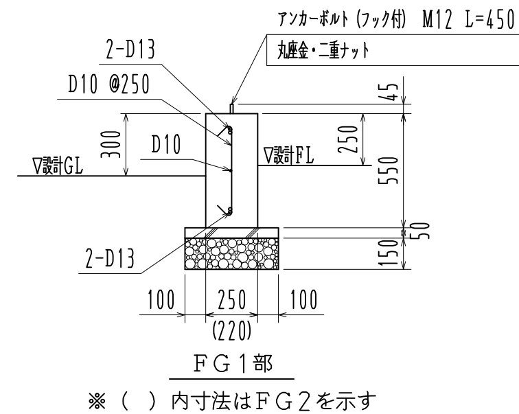
基礎詳細図 1/25
