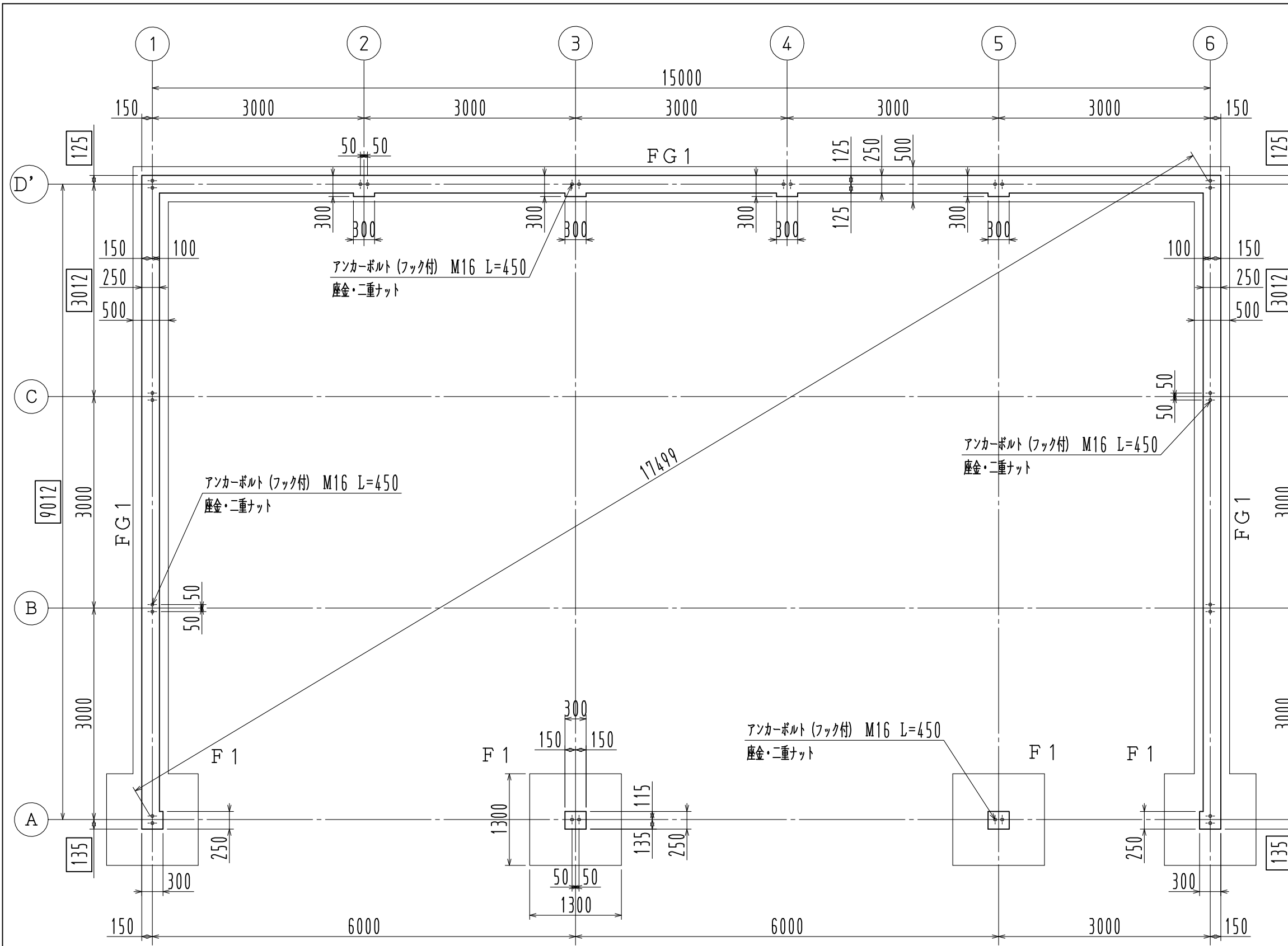
基礎伏図 1/60
