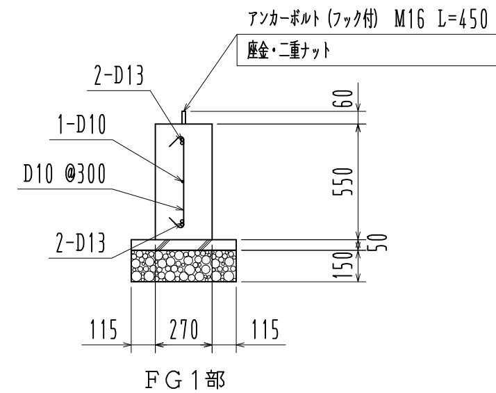
基礎詳細図 1/25
