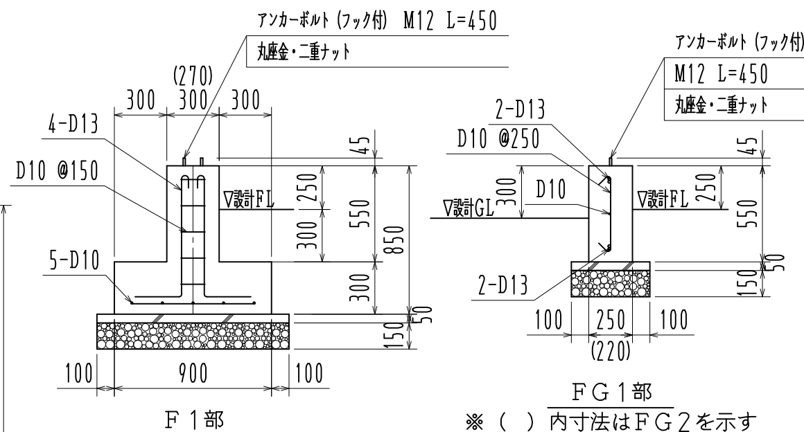
基礎詳細図 1/30
