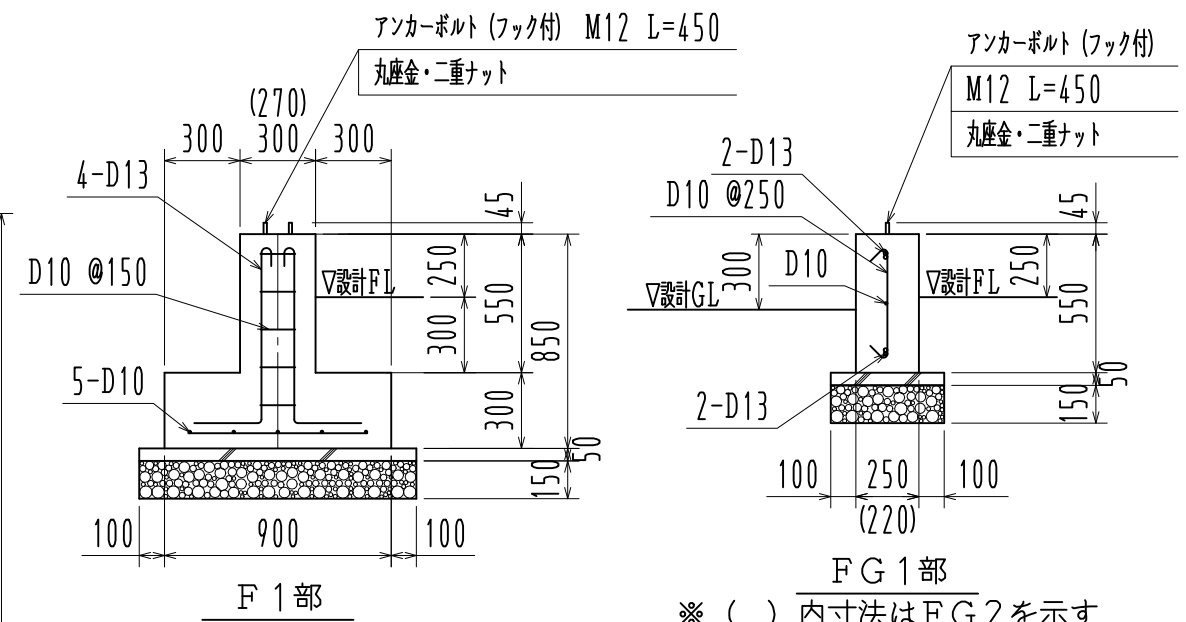
基礎詳細図 1/30
