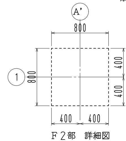
基礎詳細図 1/30
