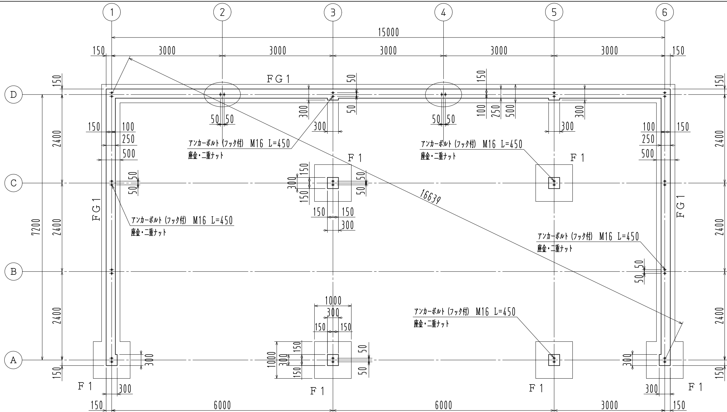
基礎伏図 1/60
