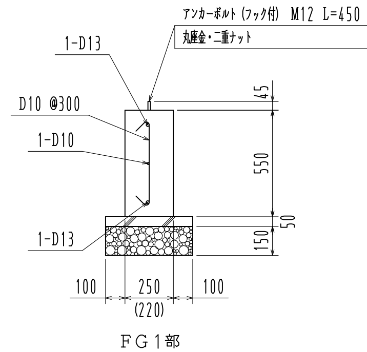
基礎詳細図 1/20
