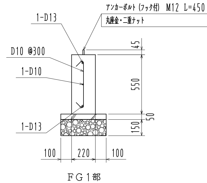
基礎詳細図 1/20
