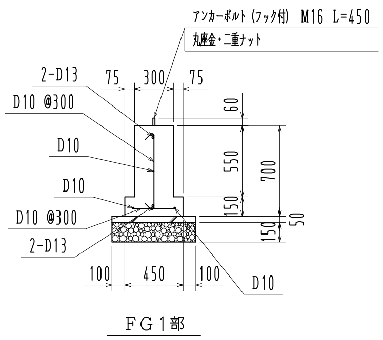
基礎詳細図 1/20
