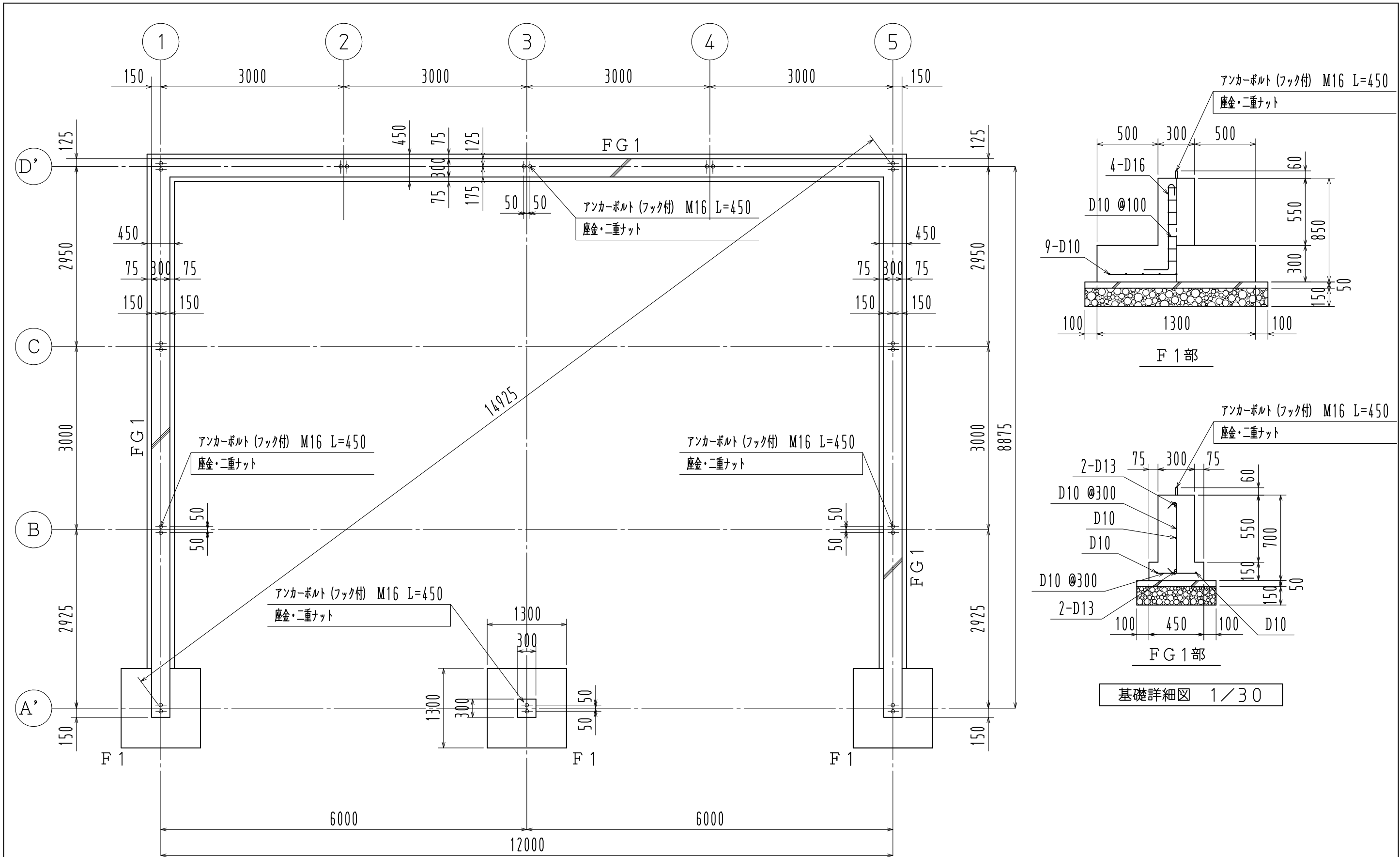
基礎伏図 1/60
