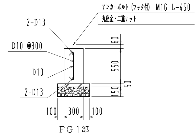
基礎詳細図 1/30
