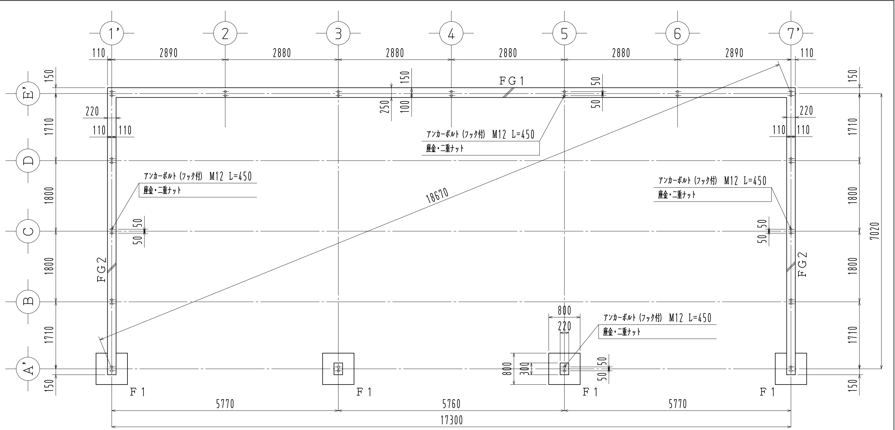
基礎伏図 1/60
