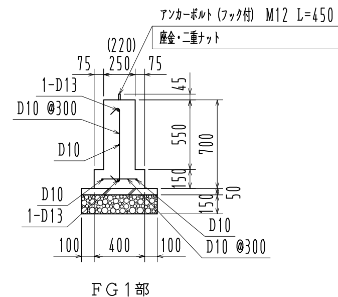
基礎詳細図 1/30
