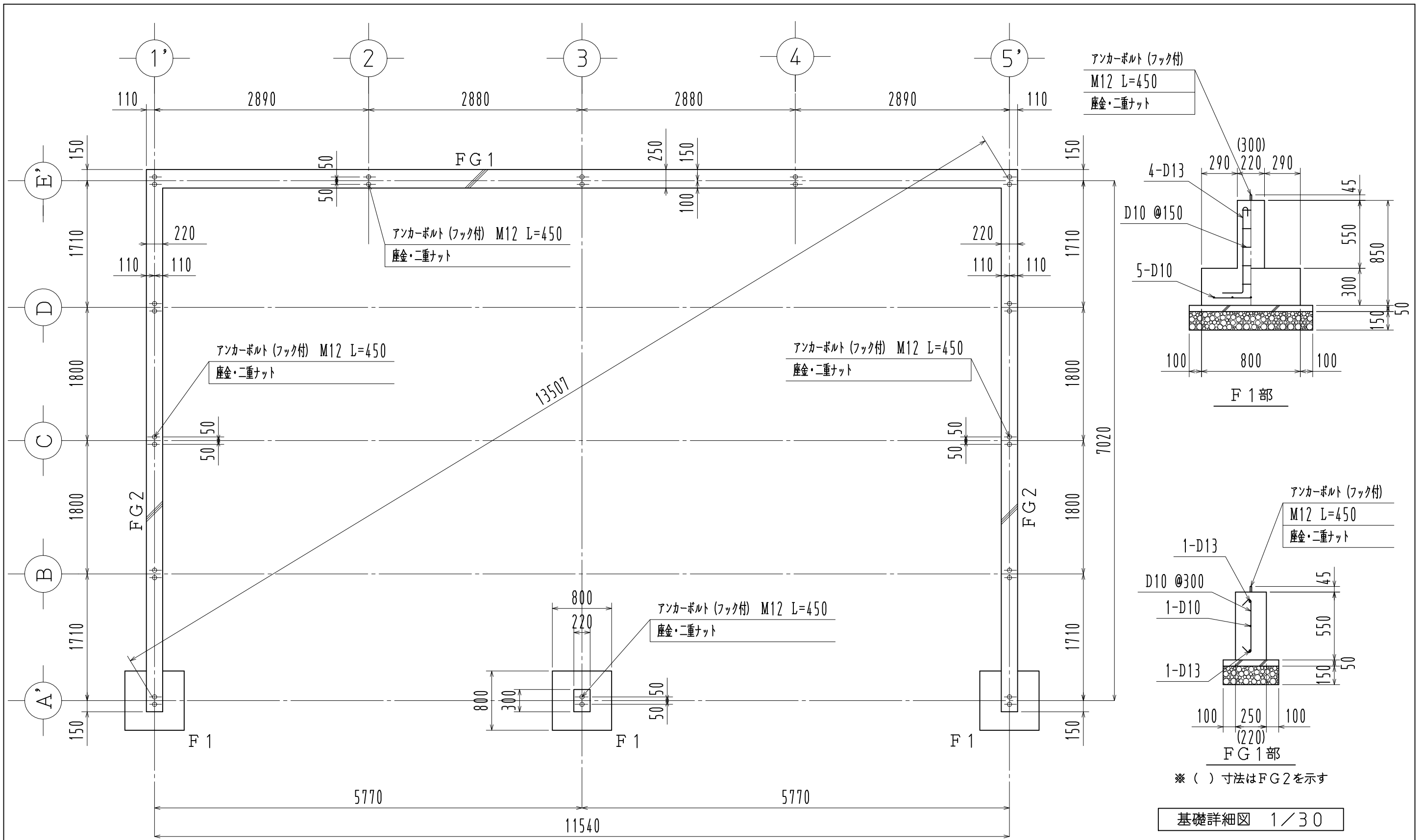
基礎伏図 1/50
