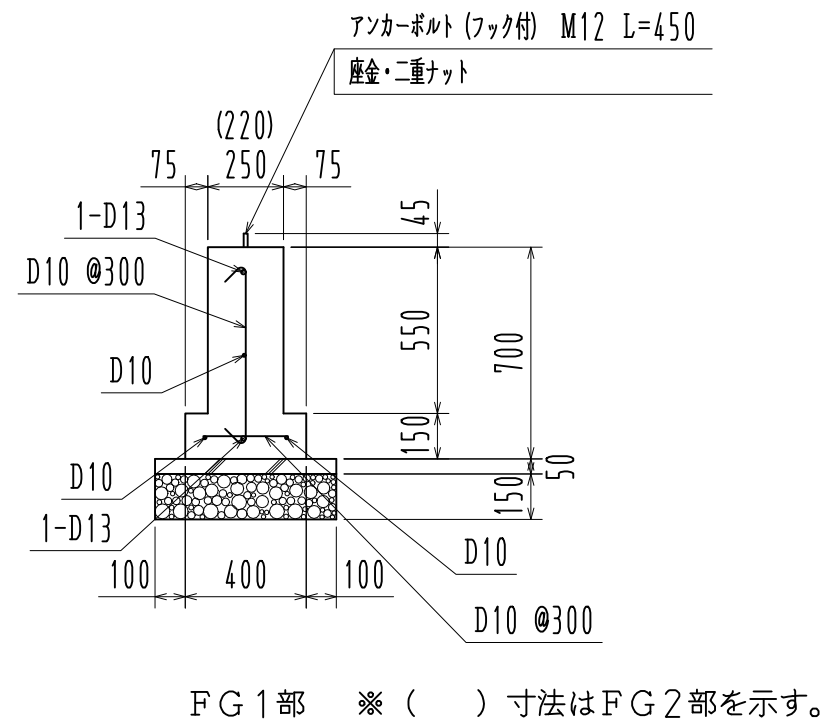
基礎詳細図 1/30
