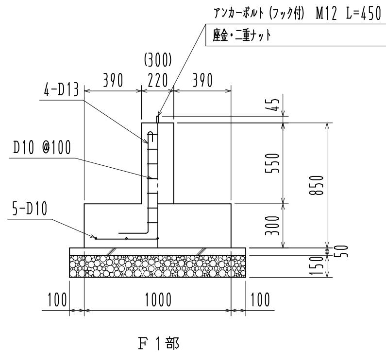
基礎詳細図 1/30
